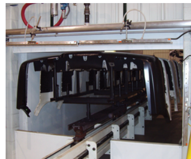
Paragolpes, carrocerías y fascias son limpiados de polvo y fibras antes del proceso de pintura.
