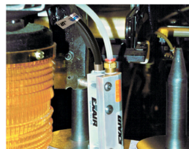
Una Cuchilla de Aire Ionizado Estándar modelo 8103 de 3" (76mm) remueve polvo de los discos duros de una computadora previo al ensamblaje.
