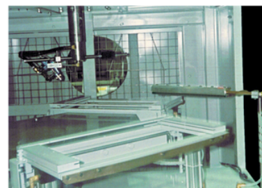
Un sistema de Cuchilla de Aire Ionizado Estándar Gen4 modelo 8212 de 12" (305mm) limpia estructuras antes de aplicarle la pintura en polvo.
