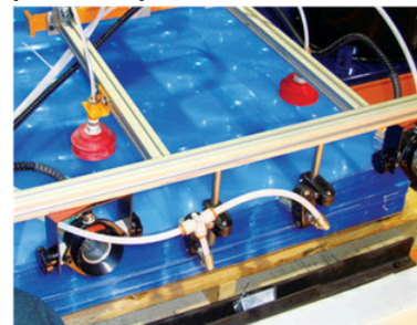
Los Cañones de Aire Ionizado Gen4 modelo 8192 proveen eliminación de estática entre los lentes de paneles solares para asistir la separación de los mismos durante la producción.
