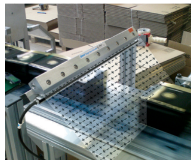
La Súper Cortina de Aire Ionizado Gen4 modelo 112118 de 18" (457 mm) elimina el polvo de productos de cuidado personal antes de sellar las cajas con celofán.
